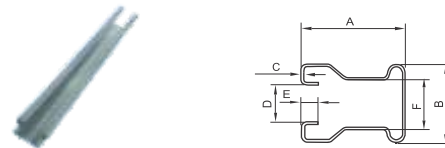
LP1005 A(mm):25 B(mm):21 C(mm):0.75 D(mm):14 E(mm):4 F(mm):14
