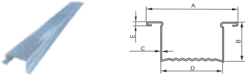
LP1003 A(mm):57 B(mm):28 E(mm):3 C(mm):0.55 D(mm):38
