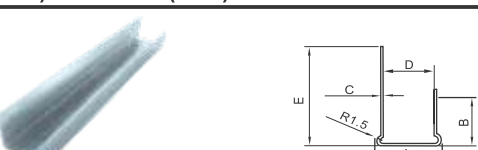
LP1020 A(mm):16.33 B(mm):13 C(mm):0.45 D(mm):12.5 E(mm):27
