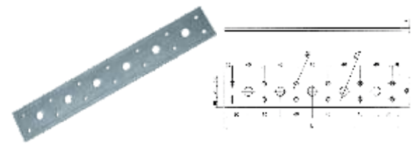
LP3018-3 T:3 L(mm):220
