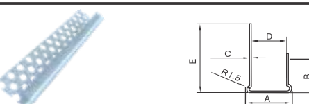
LP1018 A(mm):16.33 B(mm):13 C(mm):0.45 D(mm):12.5 E(mm):27
