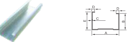
LP1010 A(mm):47 B(mm):32 E(mm):35 C(mm):0.5 D(mm):5
