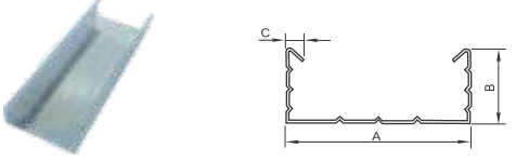
LP1006 A(mm):60 B(mm):27 C(mm):6
