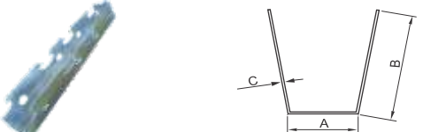
LP1008 A(mm):18 B(mm):3 C(mm):0.6
