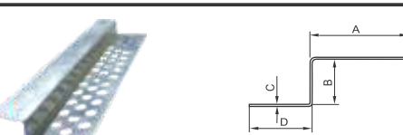
LP1016 A(mm):27 B(mm):12.5 C(mm):0.45 D(mm):17
