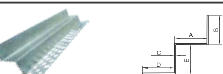
LP1017 A(mm):20 B(mm):20 C(mm):0.4 D(mm):20 E(mm):20
