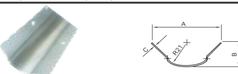
LP1021 A(mm):58 B(mm):26 C(mm):0.38
